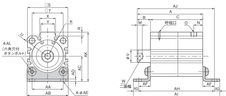
エル形寸法図
