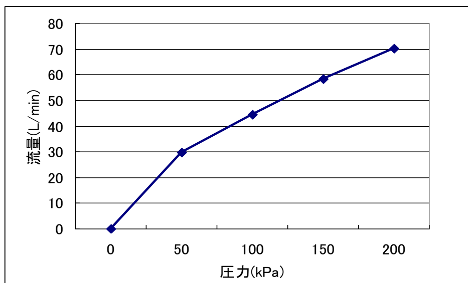
流量特性
