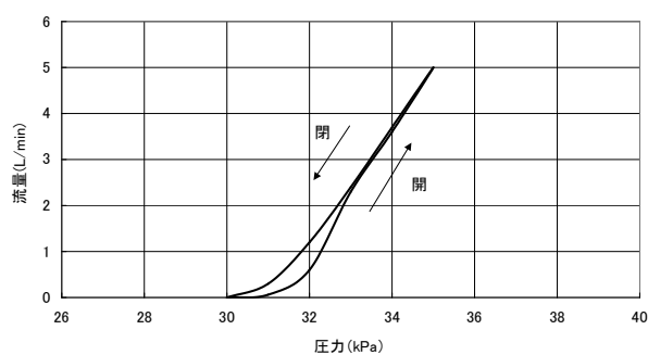
■泄压特性 ( VR1-B-M2-30 )
