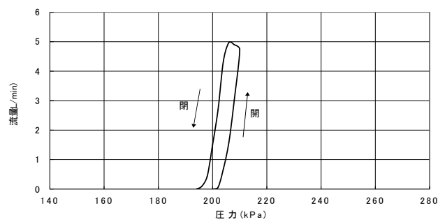
■泄压特性 ( VR1-B-M2-200 )
