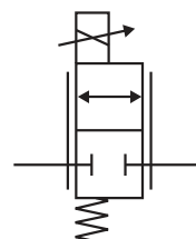
〈JIS記号〉
