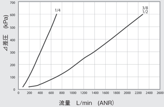
流量特性 AIR (代表値)
