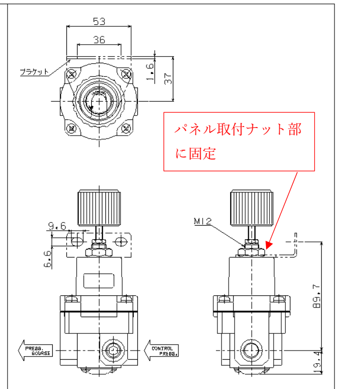
組立図 変更仕様
