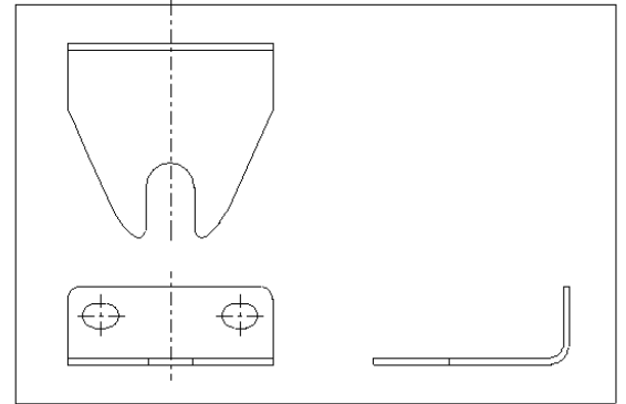
ブラケット 変更仕様
