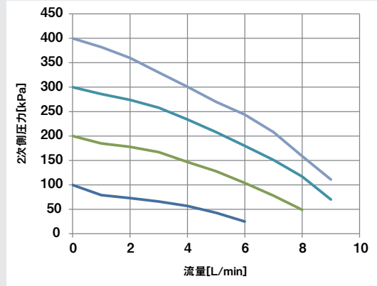
■ 流量特性
