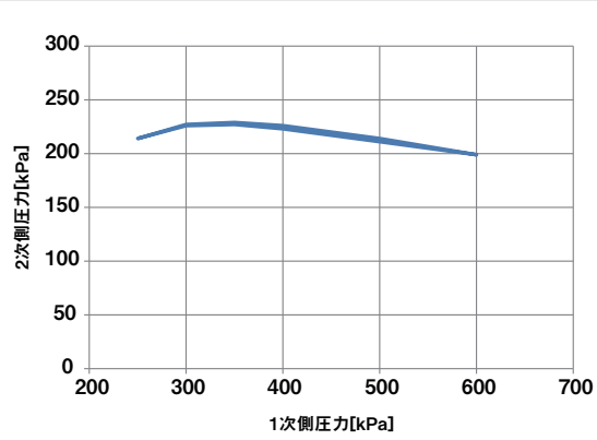
■ 圧力特性
