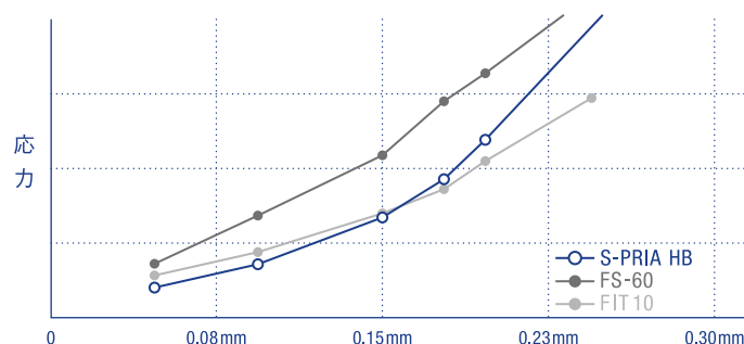
圧縮応力曲線
