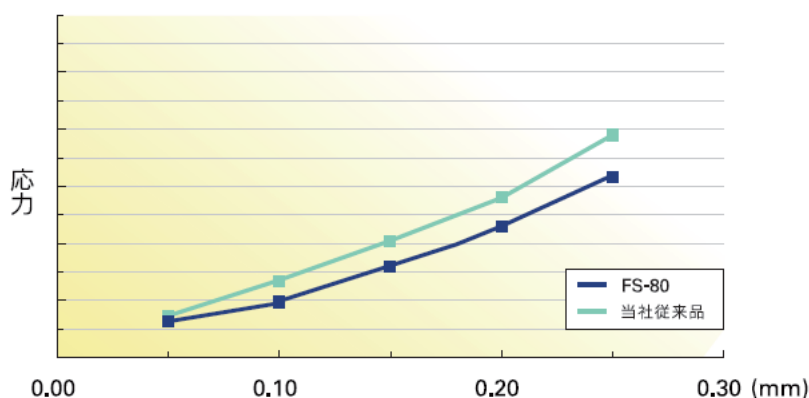
圧縮応力曲線
