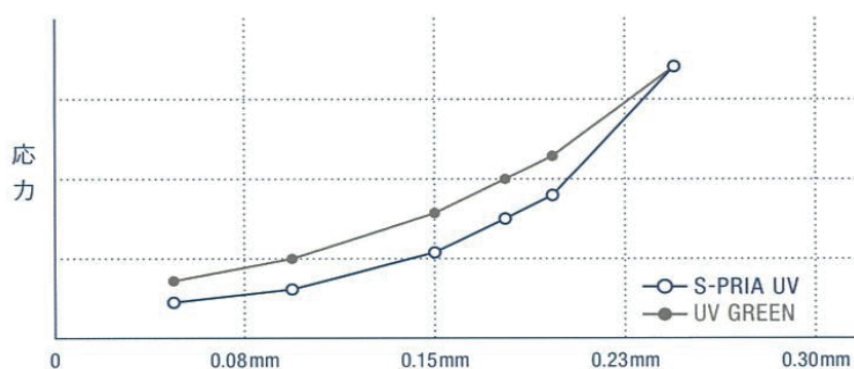
圧縮応力曲線
